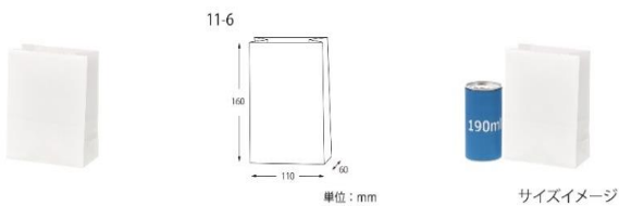
②⑤NF耐油角底袋 11-6 白無地 #004180310
