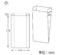
⑭NF耐油ガゼットパック 小 未晒無地 #004180201
