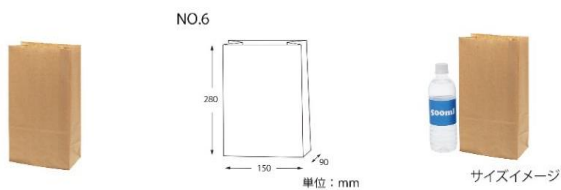
③⑫NF耐油角底袋 No. 6 未晒無地
