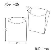
単位: mm
