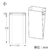
⑬NF耐油ガゼットパック 小 白無地 #004180200
